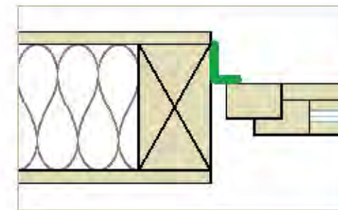
Dřevorámová konstrukce po instalaci okna Je-li okno již instalováno, nalepí se CONTEGA EXO na rám.
