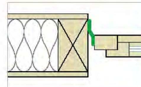
Dřevorámová konstrukce před instalací okna CONTEGA EXO již byla ze strany nalepena na rám, například firmou instalující okna.
