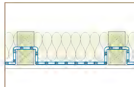
DASATOP vést pod zdvojením. Toto je stavebně fyzikálně vhodnější a šetří materiál.
