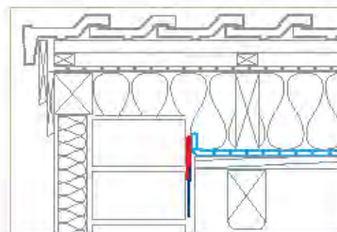
Napojení u izolace střechy shora (parobrzda např. pro clima DA)
