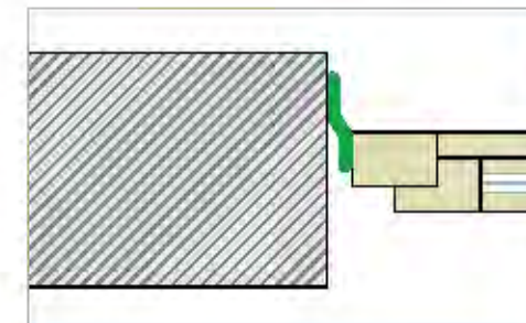
Zděná konstrukce před instalací okna CONTEGA EXO již byla ze strany nalepena na rám, například firmou instalující okna.
