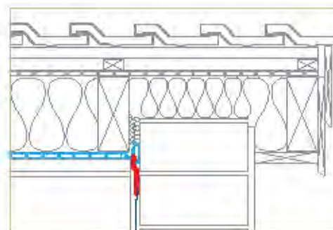
Napojení u mezikrokevní izolace (parobrzda např. pro clima DB+)
