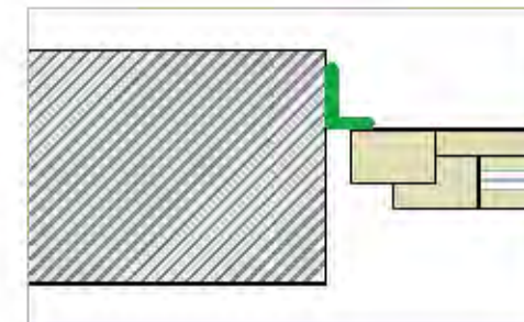
Zděná konstrukce po instalaci okna Je-li okno již instalováno, nalepí se CONTEGA EXO na rám.
