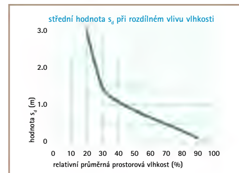
Variabilní difúzní odpor systému DASATOP je optimálně nastaven pro rychlou instalaci způsobem sub and top.
